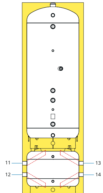
Vista B-B'
